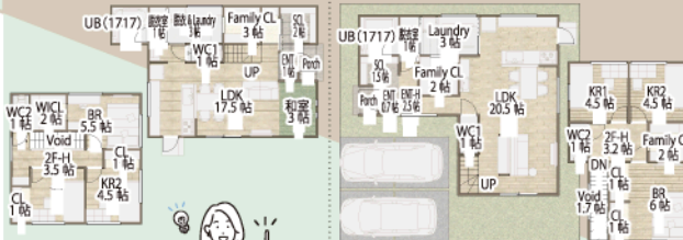
Plan21 95.2315㎡(28.81坪) 家事楽回遊動線と畳に癒される家
