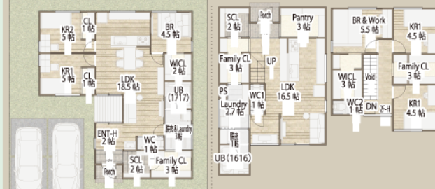
Plan45 85.2943㎡(25.8坪) インナーテラスのある家/平屋
